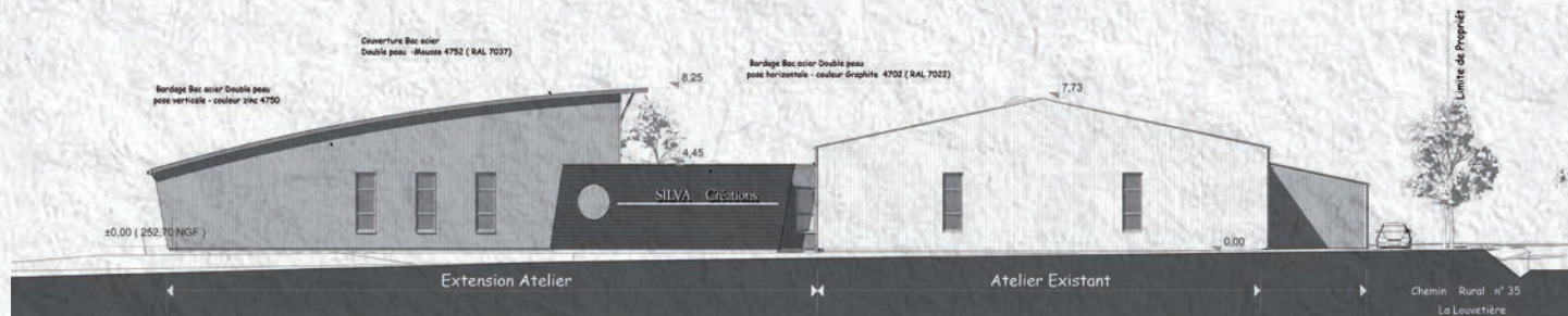
Façade Sud-Ouest
